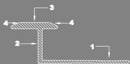
Scara 1:1 TFA117
