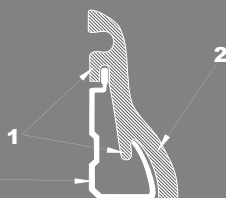
Scara 1:3 VPC505
