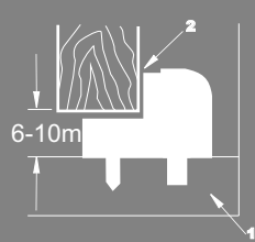
Scara 1:1 OZR442/OBR442
